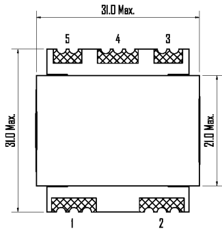
Dimensions (Unit:mm)
